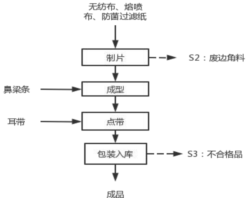
图 2-5 一次性医用口罩生产工艺流程图
