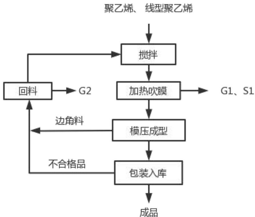
图 2-4 医用手套生产工艺流程图
